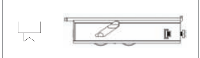
01-551BL – Impact Door Stop
